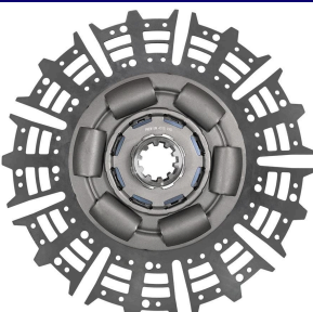
MB 1935 O 400 10 ESTRIAS 6 MOLAS 430MM (SACHS 5697)
