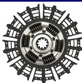
VW METEOR 28.460 / 29.530 MAN 6 MOLAS 10 ESTRIAS 430MM (SACHS 5581)
