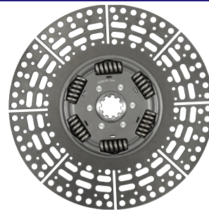
VW TITAN SEM PRÉ DAMPER 6 MOLAS 10 ESTRIAS 380MM (SACHS 5080)
