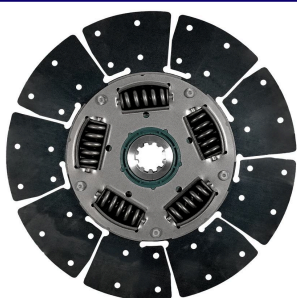
FORD CARGO 350MM (SACHS 5266)
