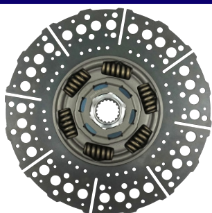
MB 1418 6 MOLAS 18 ESTRIAS 362MM (SACHS 5523)
