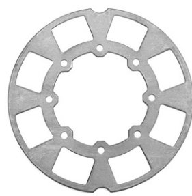
CHAPA REFORÇADA EATON 365MM 8 MOLAS
