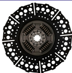
IVECO VERTIS 10 ESTRIAS 6 MOLAS 362MM
