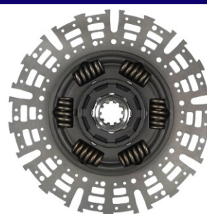
VW TGX MAN 6 MOLAS 10 ESTRIAS 430MM (SACHS 5705)
